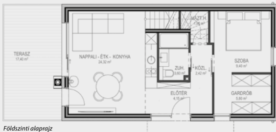
Földszinti alaprajz
