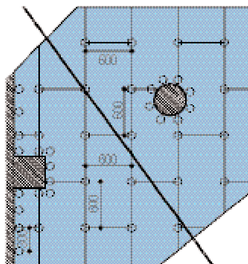
Lábelhelyezés álpadlót áttörő szerkezet körül
