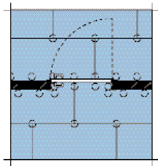
Álpadló megerősítése lábsűrítéssel az ajtónál
