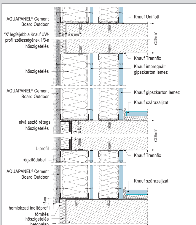
W387E-V1 Metszet
