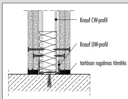
W382-VU1 Ajzatcsatlakozás
