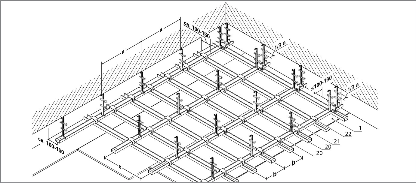
Átnézeti rajz
