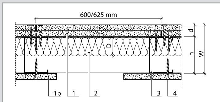
El 30 aknafal, alaprajz
