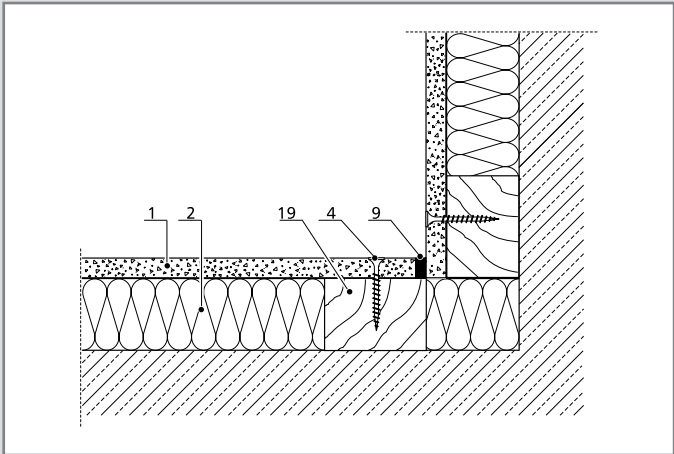
Negatív sarokkialakítás
