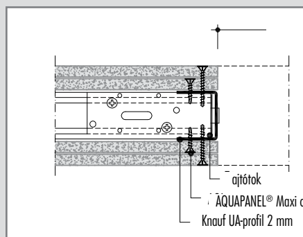
W382-E1 Nyílás kialakítás UA profillal
