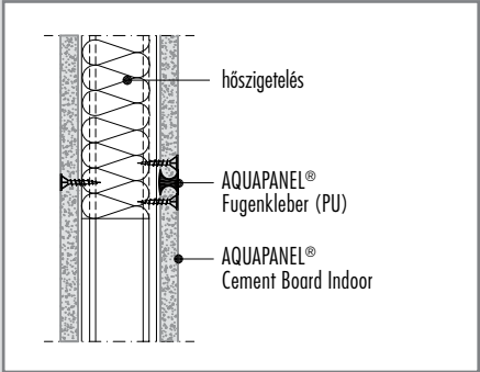
W381-C1 T-csatlakozás
