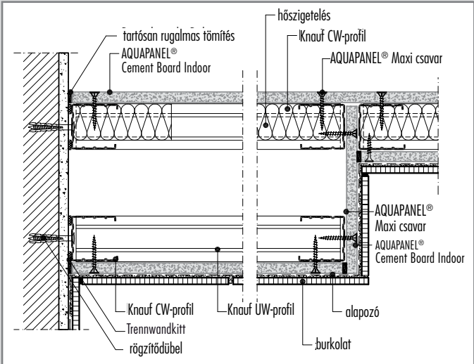
W386-VA1 Csatlakozás hagyományos falszerkezethez
