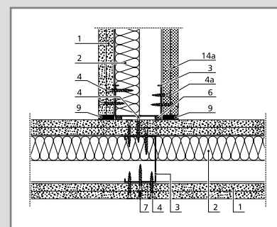
T-csatlakozás
