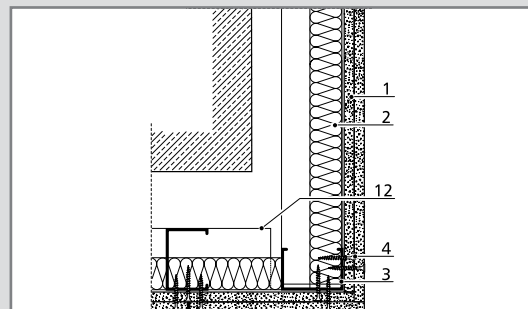
Pozitív sarokkialakítás
