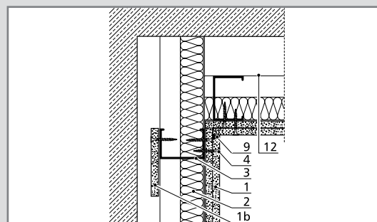
Negatív sarokkialakítás
