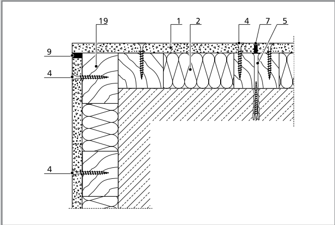
Pozitív sarokkialakítás
