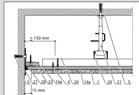
Árnyékfuga kialakítás
