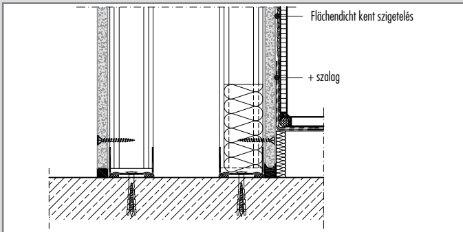
W386-VU1 Aljzatcsatlakozás
