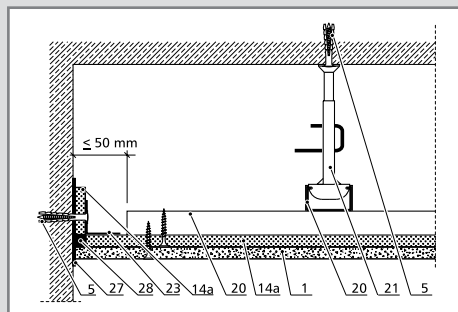
Álmennyezet-falazat csatlakozás tűzvédelmi követelmény esetén
