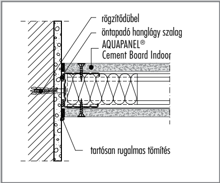
W381-A1 Hagyományos falcsatlakozás
