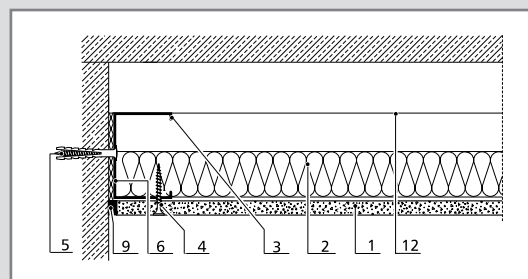
Csatlakozás falazathoz
