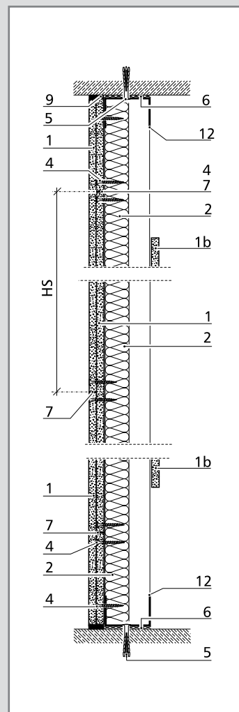
El 30 aknafal, metszet
