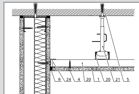
Válaszfal-álmennyezet csatlakozás tűzvédelmi követelmény nélkül
