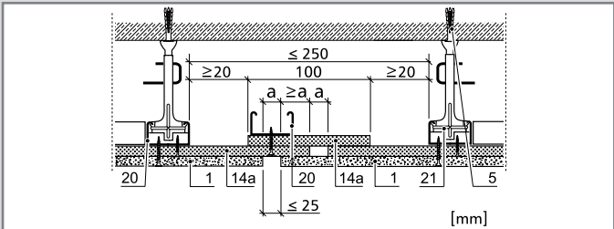
Mozgási hézag tűzvédelmi követelmény esetén
