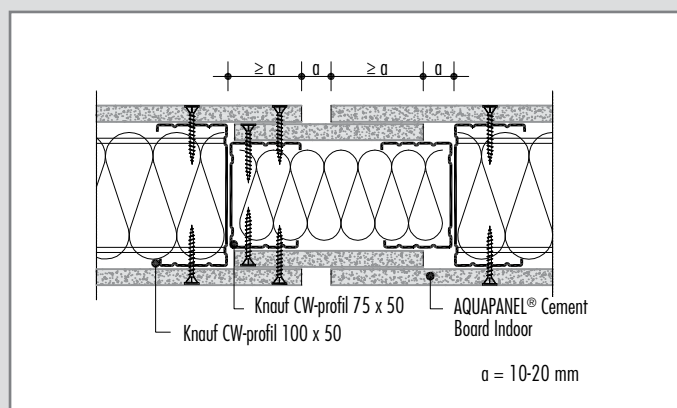
W381-BFU1 Mozgási hézag EI 30
