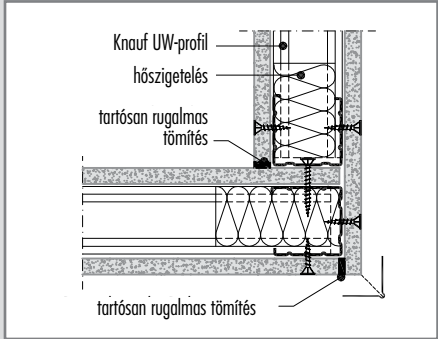
W381-D1 Sarokkialakítás
