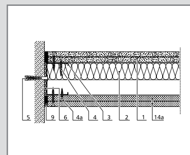
Csatlakozás falazathoz
