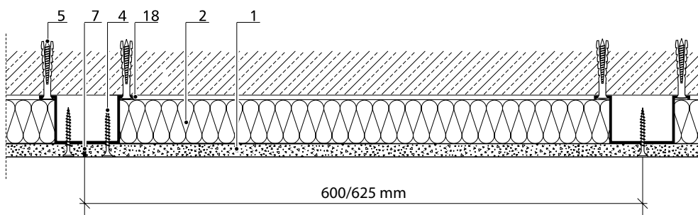
Rögzítés akusztikus lengőkengyellel, kalaprofillal vagy közvetlen felfüggesztővel
