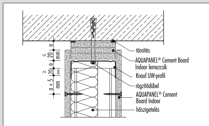
W381-V03 Csúszó födémkapcsolat
