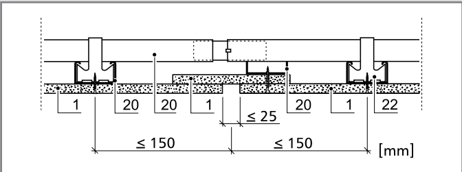
Mozgási hézag
